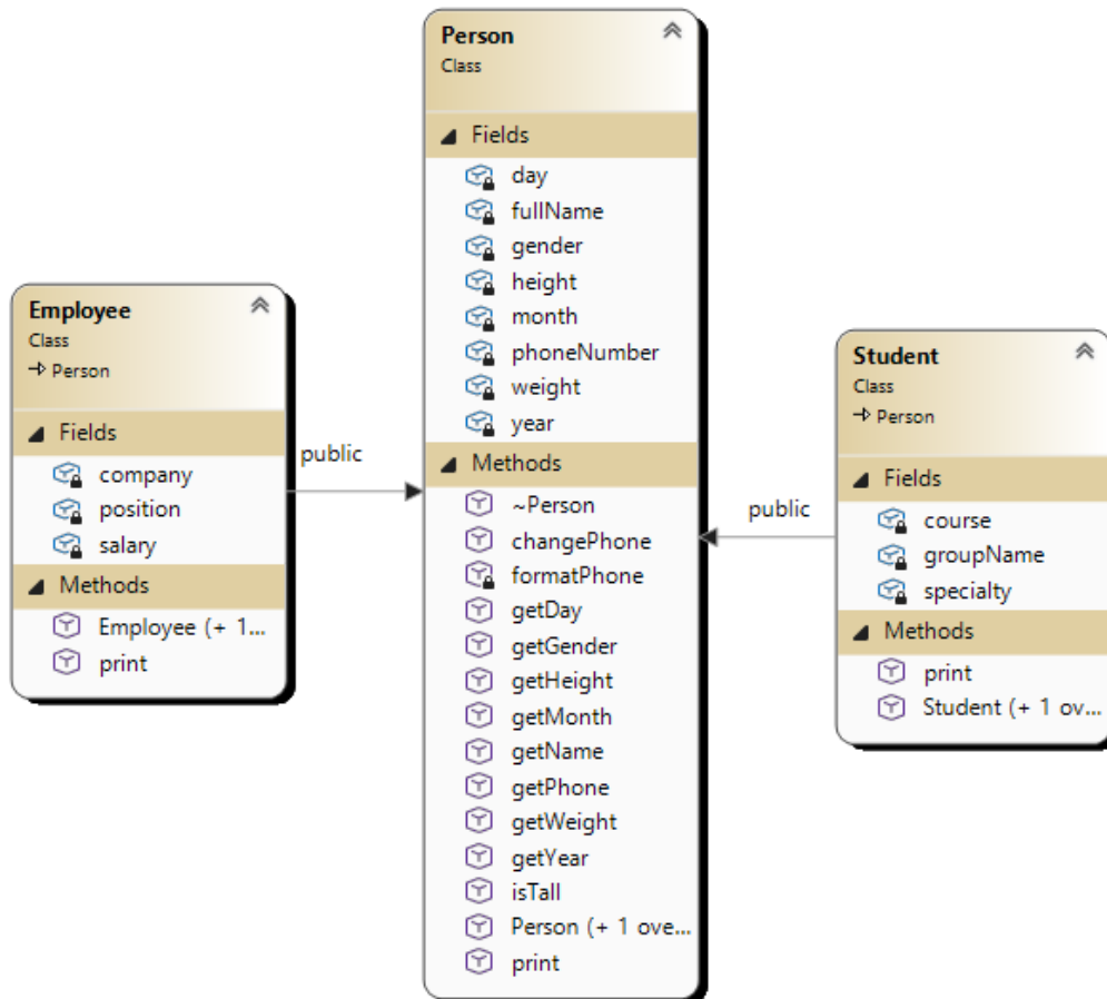
Рисунок А1. – Діаграма класів
